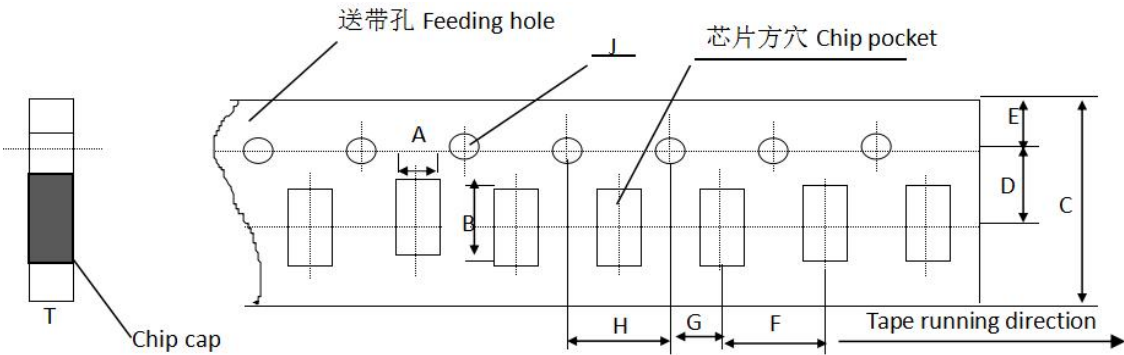
纸带运行方向
